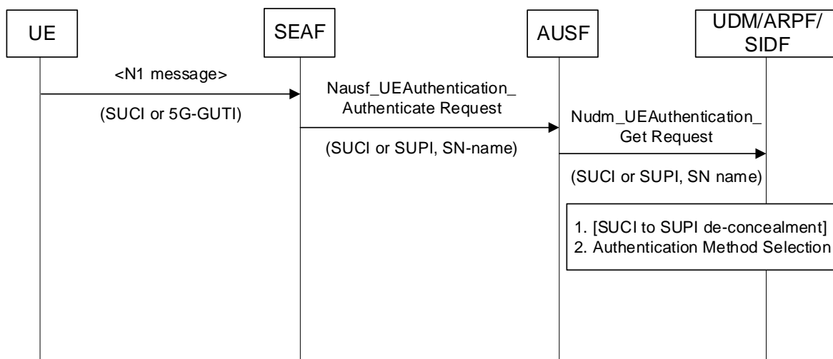
Рисунок 4.7 – Запуск процедуры аутентификации
