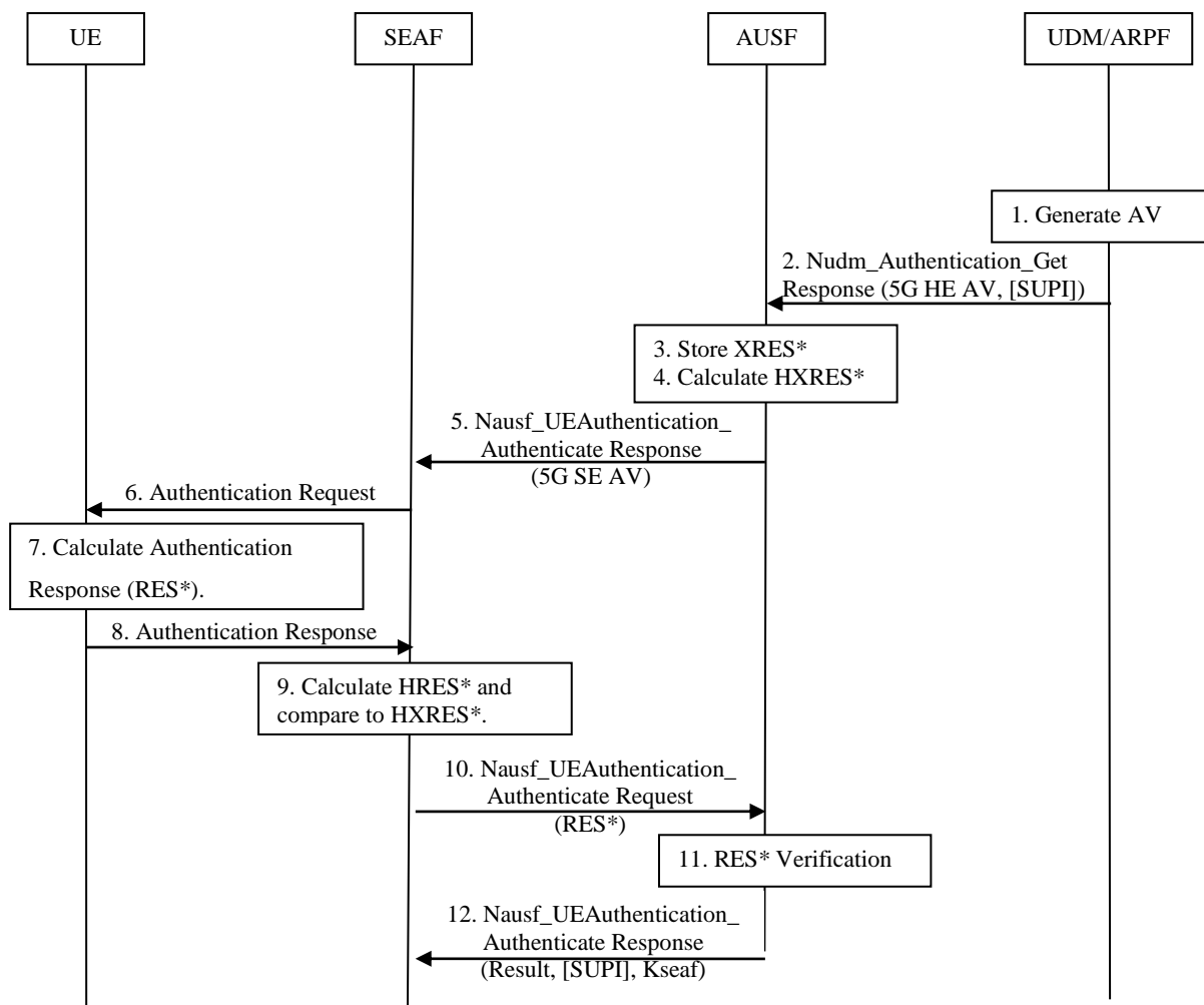
Рисунок 4.8 – Процедура аутентификации по алгоритму 5G-AKA
