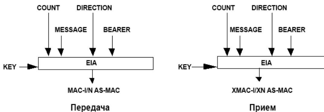
Рисунок 3.11 – Алгоритм проверки целостности в E-UTRA
