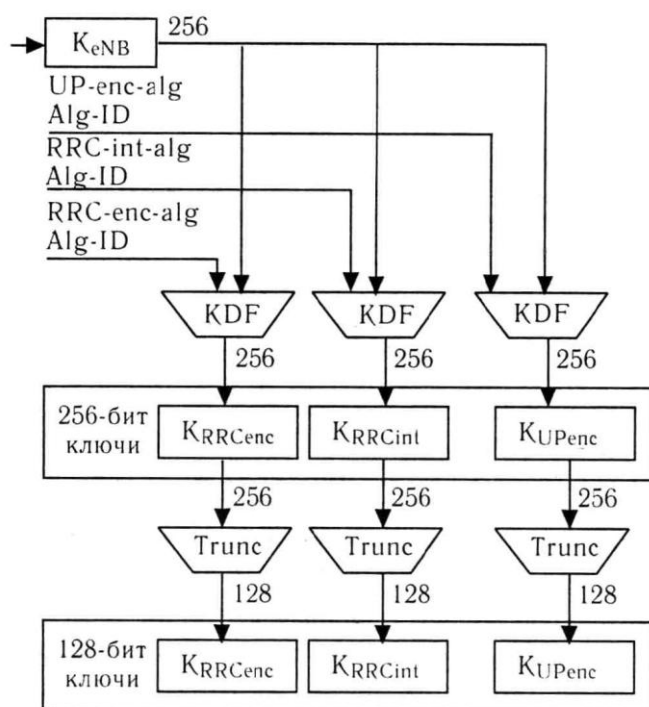
Рисунок 3.8 – Генерирование ключей для сигнализации AS и пакетов трафика UP
