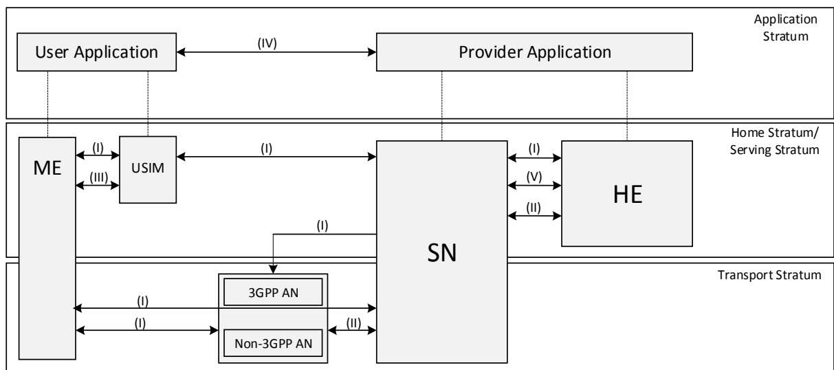
Рисунок 4.3 – Базовая структура безопасности в сетях 5G
