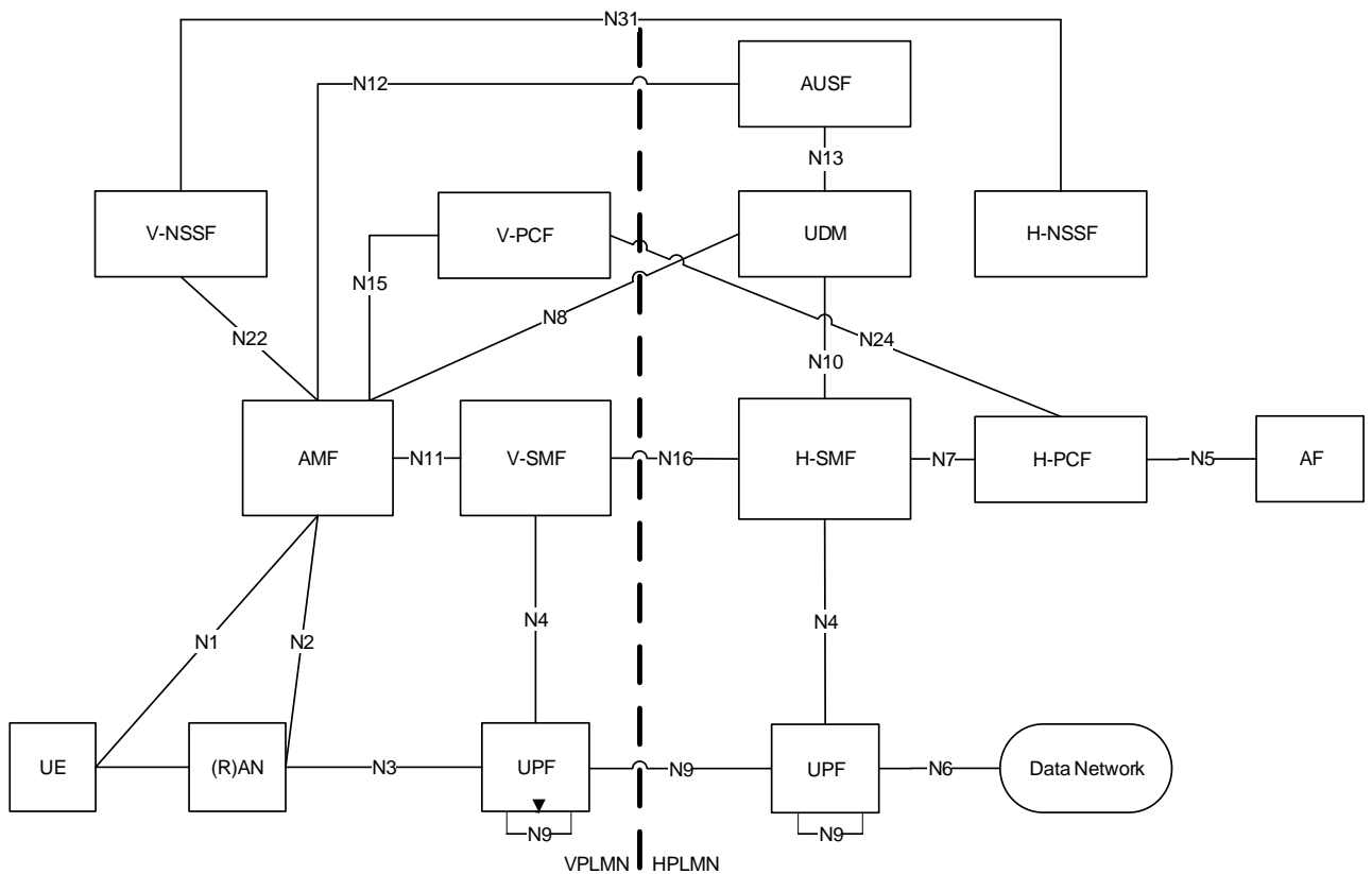
Рисунок 4.2 – Архитектура NR при роуминге при доставке трафика через домашнюю сеть
