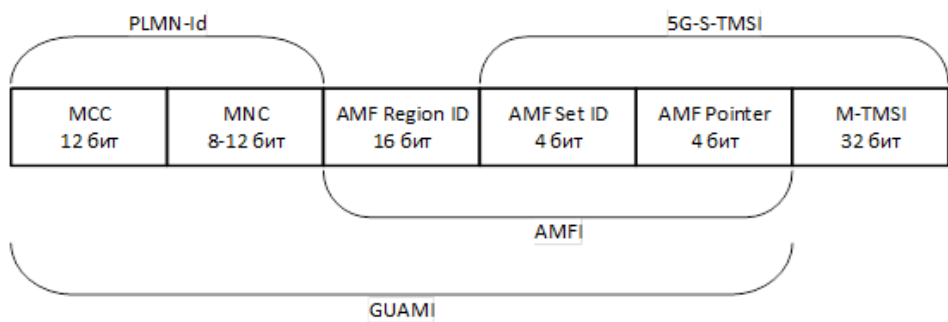
Рисунок 4.6 – Формат 5G-GUTI
