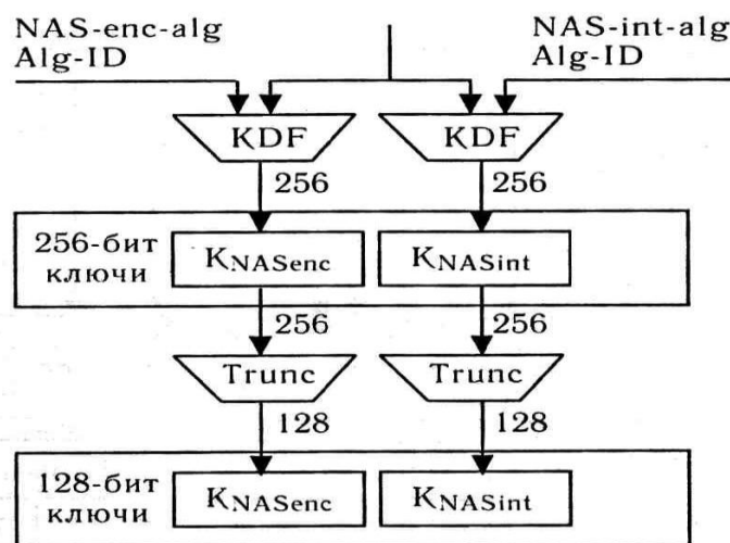
Рисунок 3.7 – Генерирование ключей шифрации и целостности для NAS сигнализации
