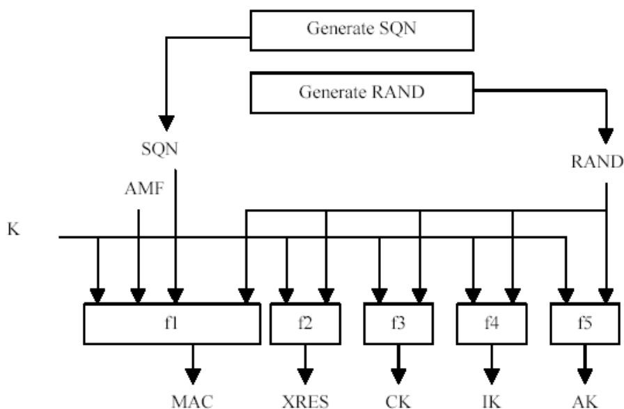
Рисунок 3.3 – Исходный алгоритм генерации вектора аутентификации
