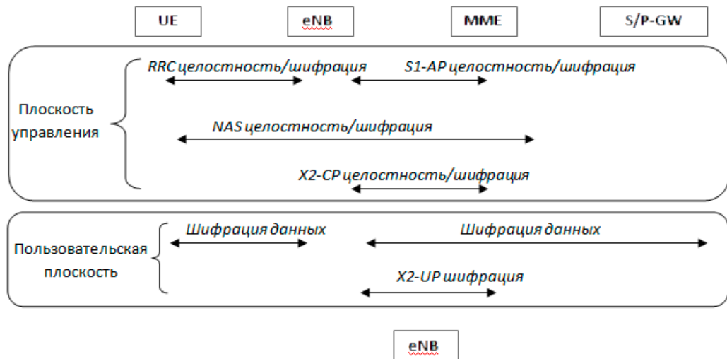
Рисунок 3.9 – Реализуемые процедуры безопасности в сети E-UTRAN
