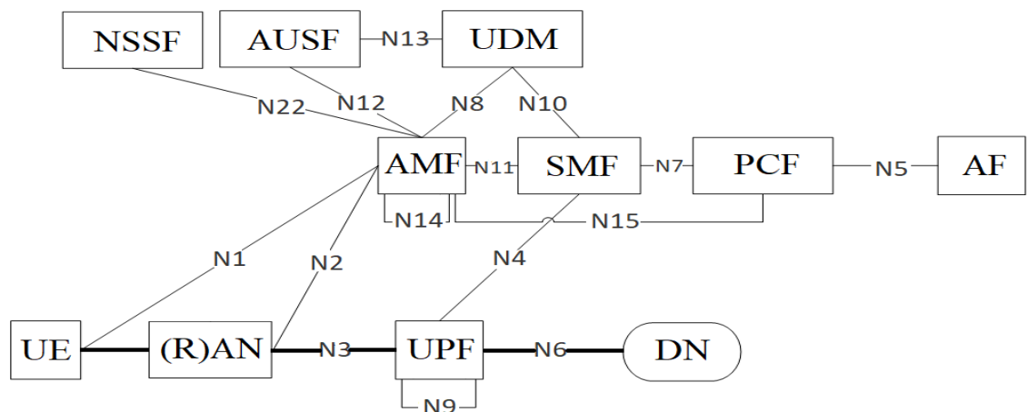
Рисунок 4.1 – Архитектура NR
