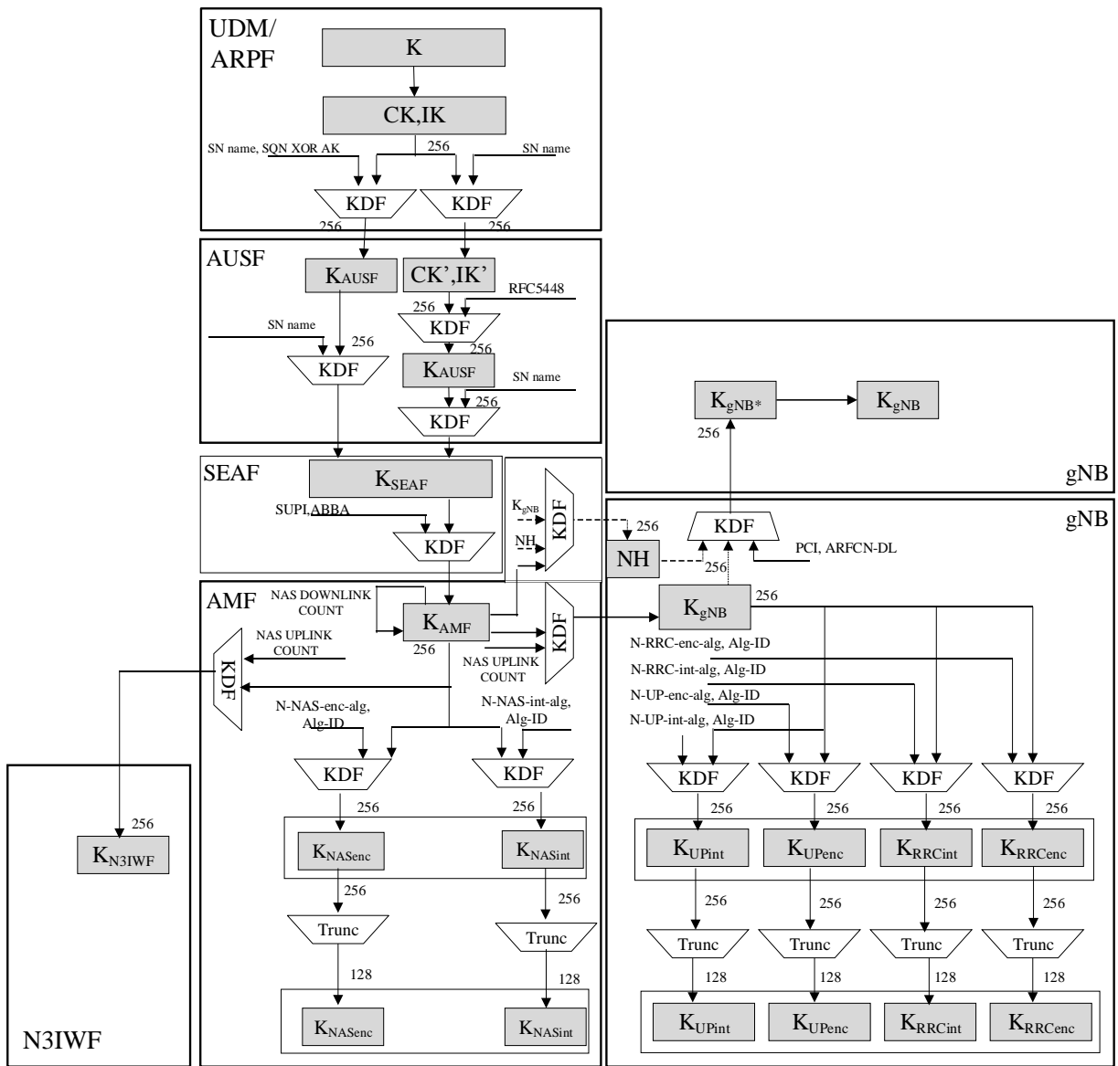
Рисунок 4.10 – Генерация ключей для UE
