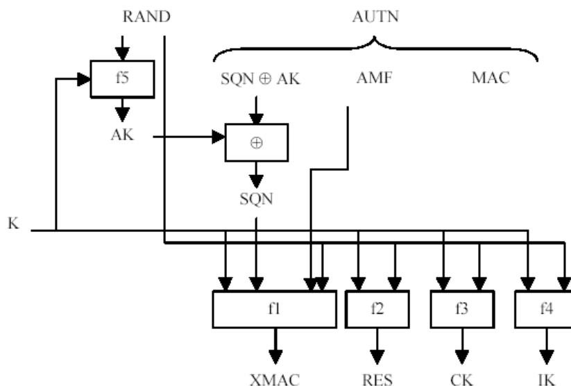
Рисунок 3.5 – Процедура аутентификации в USIM
