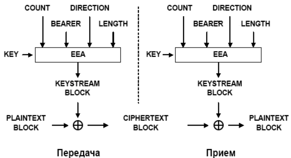
Рисунок 3.10 – Алгоритмы шифрации и дешифрации в E-UTRAN
