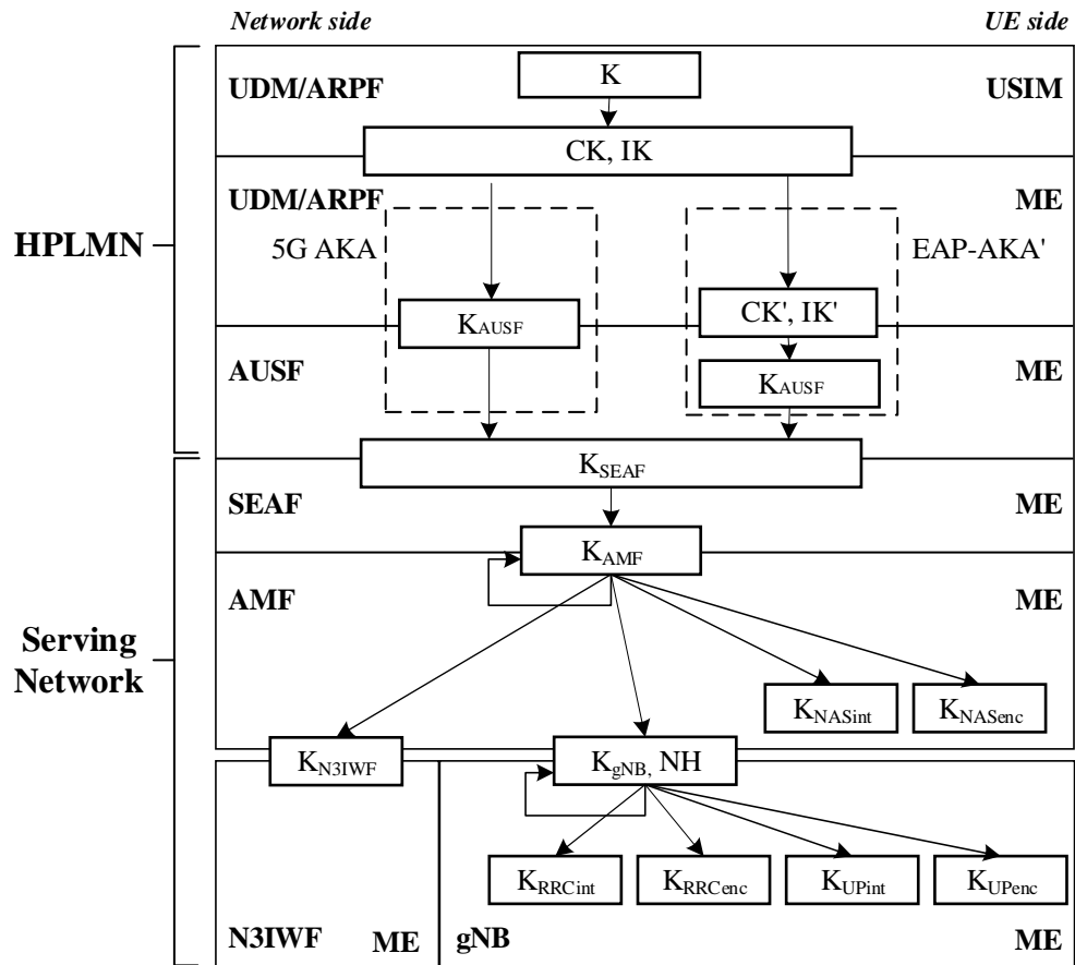
Рисунок 4.9 – Иерархия ключей в 5G NR
