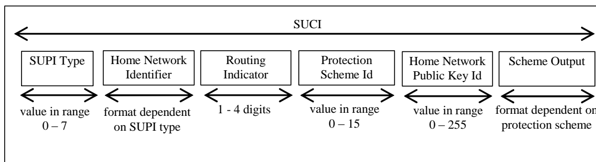
Рисунок 4.5 – Структура SUCI
