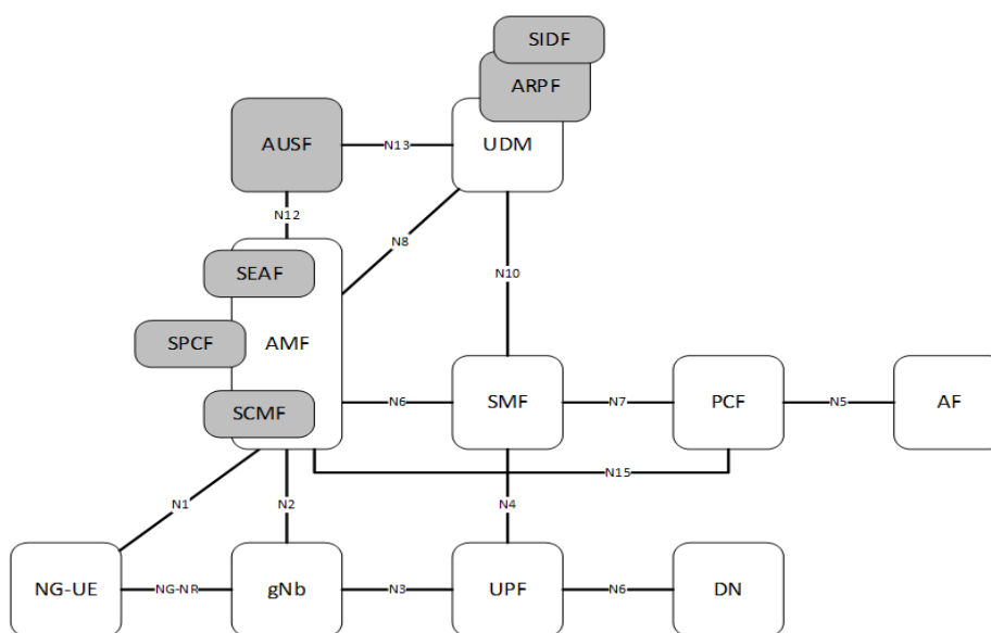
Рисунок 4.4 – Общая архитектура построения ядра сети 5G
